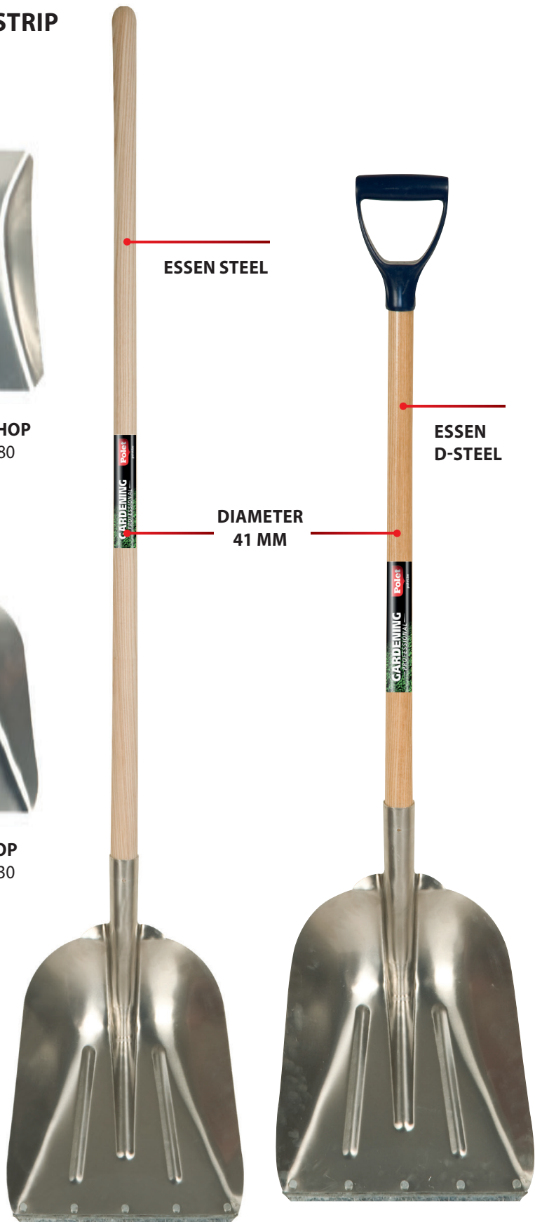
GRAANSCHOP • 410 x 330 mm • 500 x 360 mm
